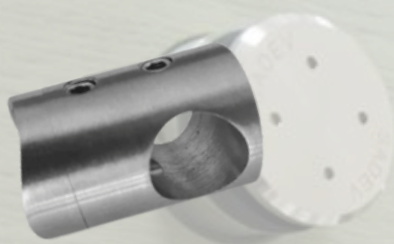
CONECTOR A POSTE BASE CURVA PARA TUBO DE 50.8MM
