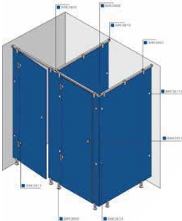
Diagrama herrajes para baño cuadrado
