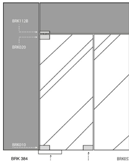
Herraje superior para punto de giro superior. Acabado: Negro Mate.
