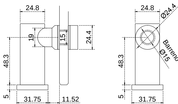
GLR 676C
