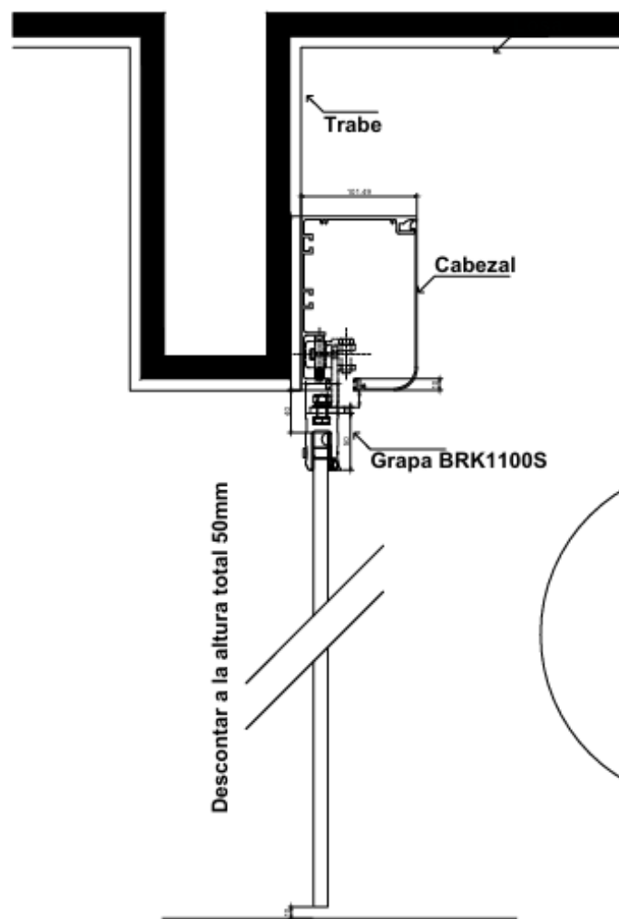
Detalle cabezal sistema automático
