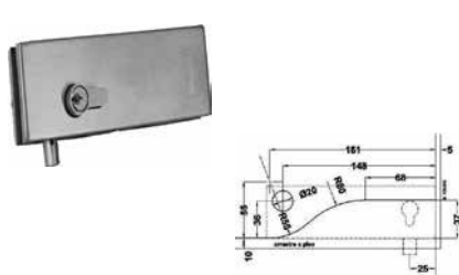
Chapa a piso con resaque. Acabado: Satín y cromo.
