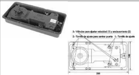
Bisagra hidráulica para 120 kg. Material cubierta: Acero inoxidable. Acabado: Satín. Medidas: Perforación de piso 145 x 299 x 50 mm.
