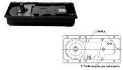
Bisagra hidráulica para 80 Kg. Medidas para perforación a piso: 100 x 266 x 51 mm.
