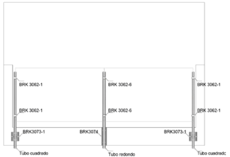
Diagramas de simulación para acomodo de herrajes para barandal.
