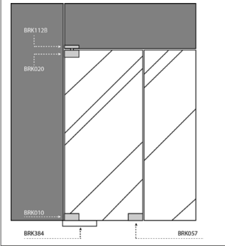
Herraje superior para punto de giro superior. Acabado: Satín y cromo.
