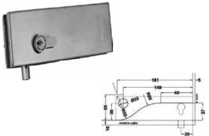
Chapa a piso con resaque. Acabado: Satín y cromo.
