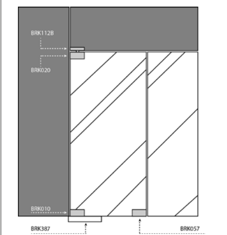
Herraje superior para punto de giro superior. Acabado: Satín y cromo.
