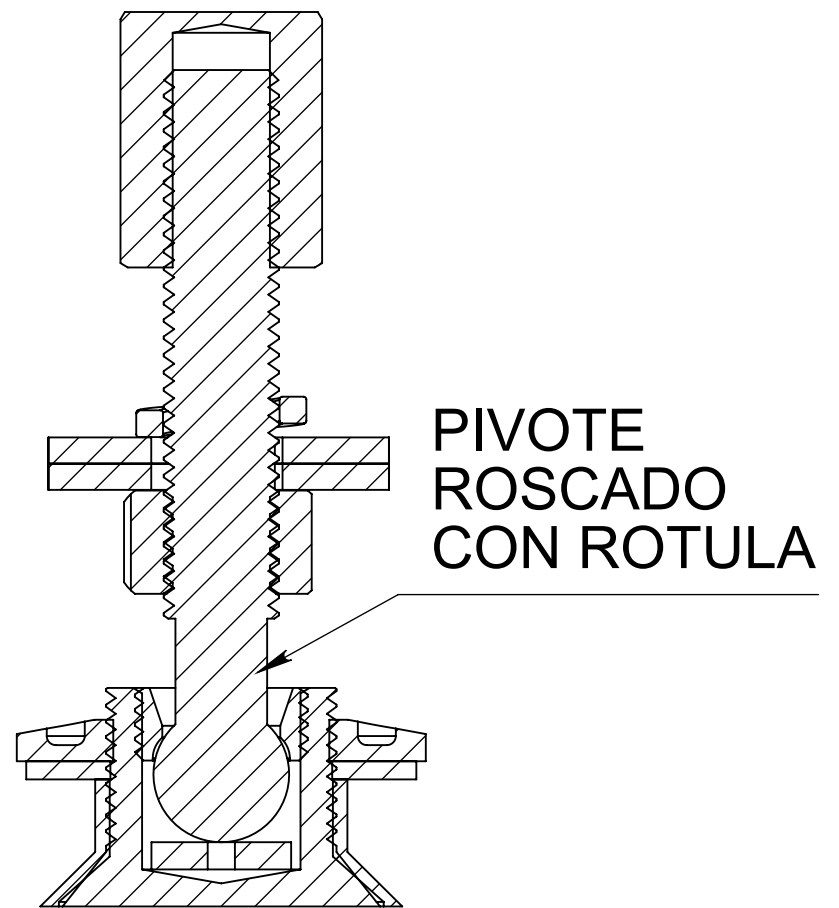
SECCIÓN A-A ESCALA 1.2 : 1
