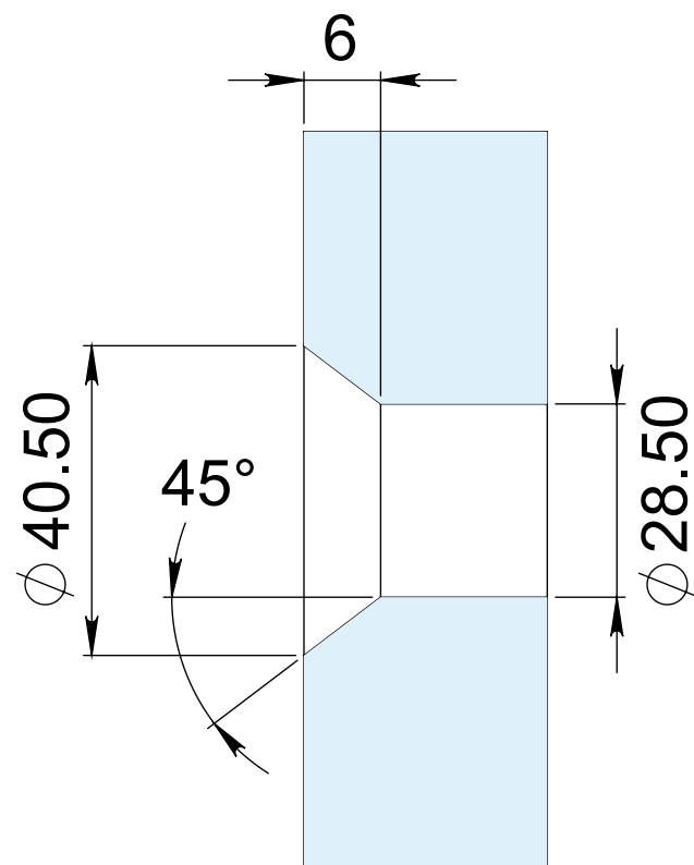
BARRENADO EN VIDRIO
